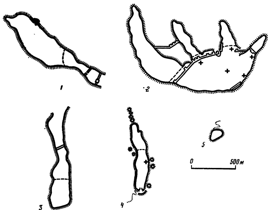
Рис. 3. Планы средневековых крепостей бассейна р. Качи и других «пещерных городов» Крыма.
